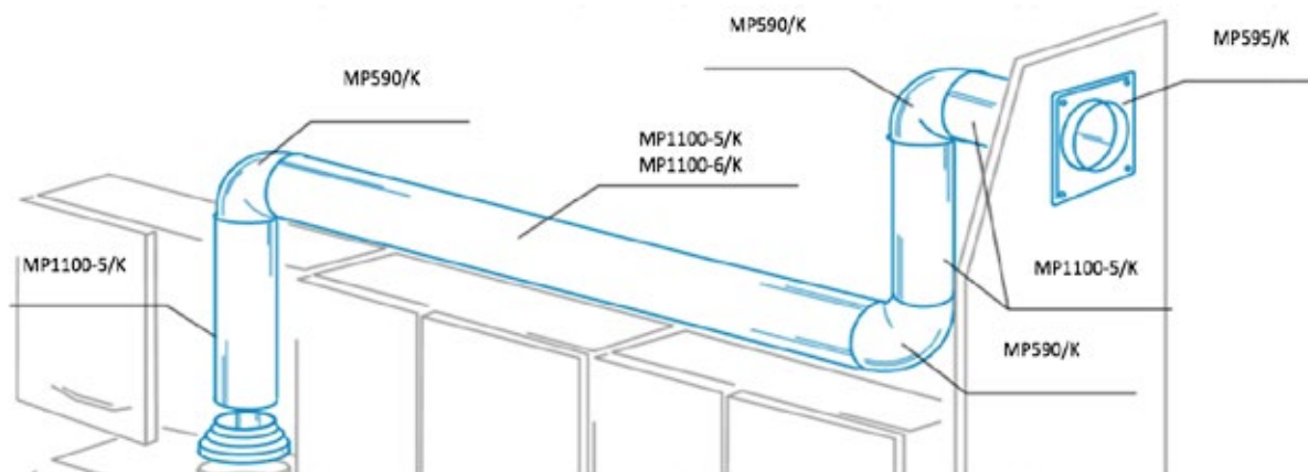
PŘÍKLAD INSTALACE - KULATÉ POTRUBÍ
