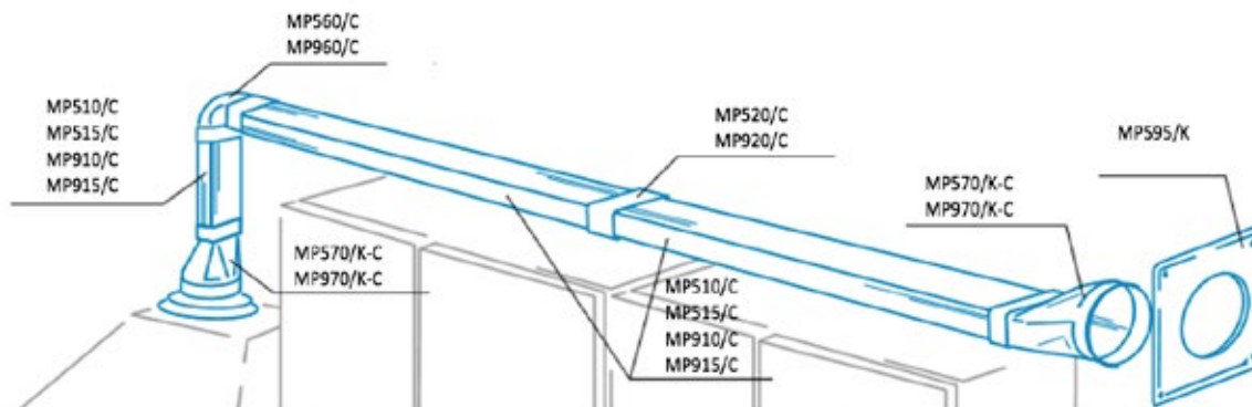
PŘÍKLAD INSTALACE - PLOCHÉ POTRUBÍ
